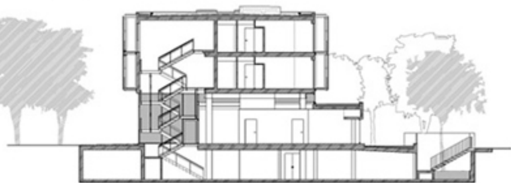
sezione trasversale/transversal section
