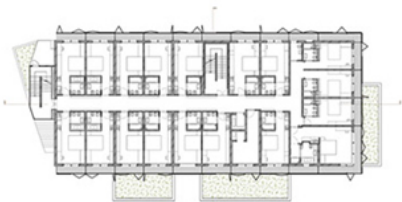
pianta del primo e del secondo piano/layout of the first and second floors
